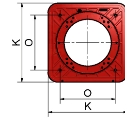
Plantilla de perforación de la placa de la caldera.
