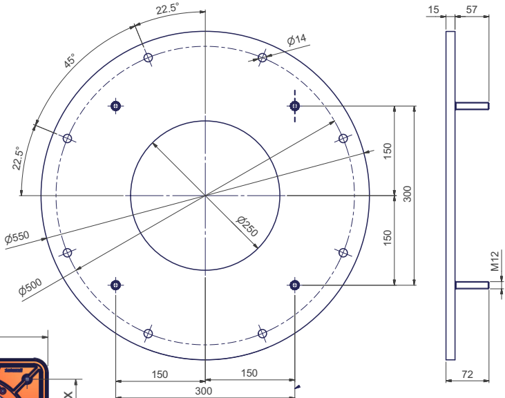
Brida de adaptación aconsejada
