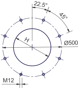
Plantilla de perforación recomendada de la placa de la caldera.
