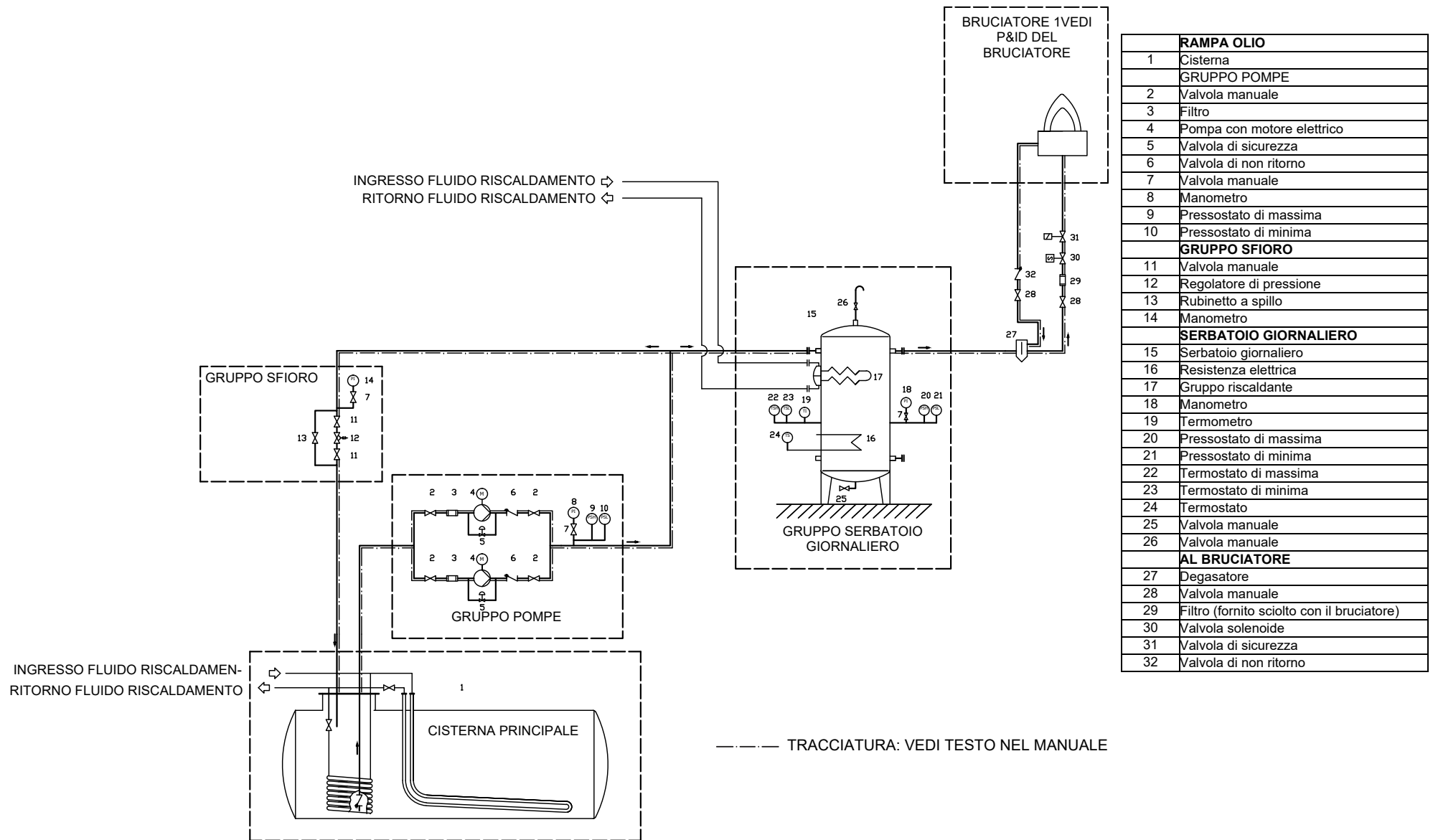
Fig. 12 - 3ID0023 v2 - Schema idraulico - Configurazione per un solo bruciatore
