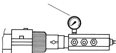
Inserimento manometro
