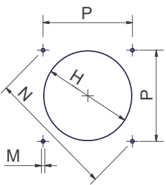
Plantilla de perforación recomendada de la placa de la caldera.
