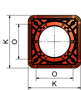
Фланец горелки
