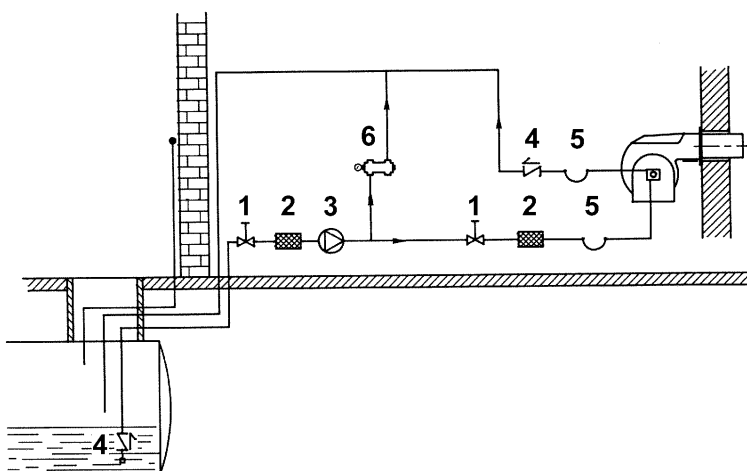
Рис. 6 - Кольцевой контур подачи топлива
