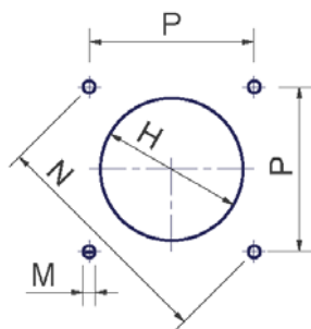
Рекомендуемая амбразура котла (RG1025 / RG1030)
