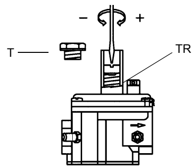
Стабилизатор давления
