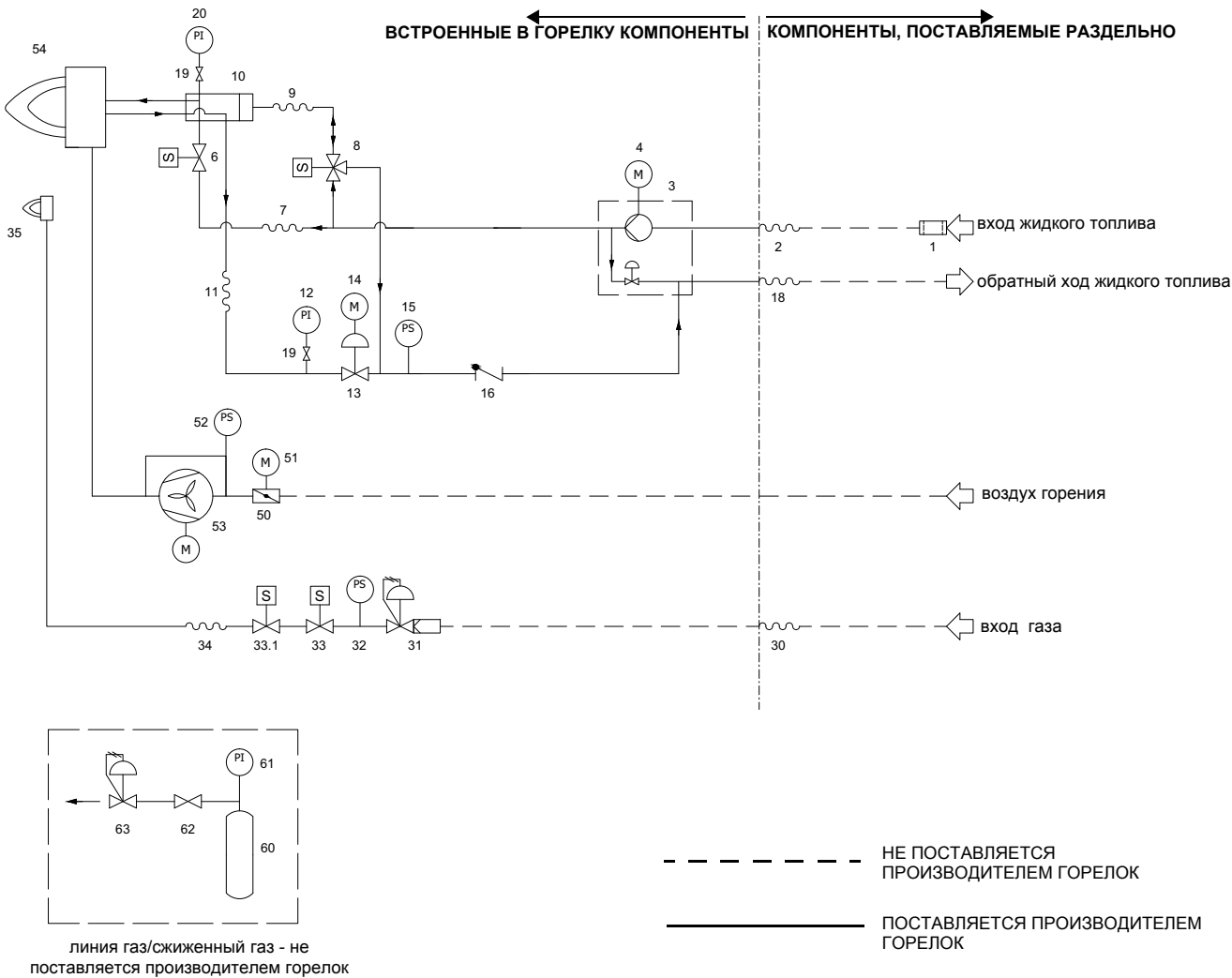
Рис. 2 - 3I2G-27 v0 – Гидравлическая схема для форсунки типа M3
