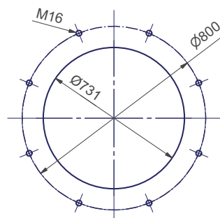
Рекомендуемая амбразура котла (RG1040)
