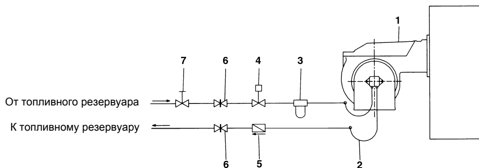
Рис. 4 - Двухтрубная система
