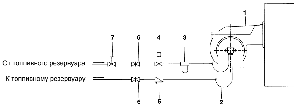
Рис. 4 - Двухтрубная система
