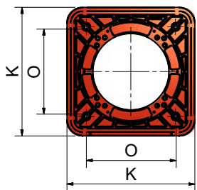
Фланец горелки
