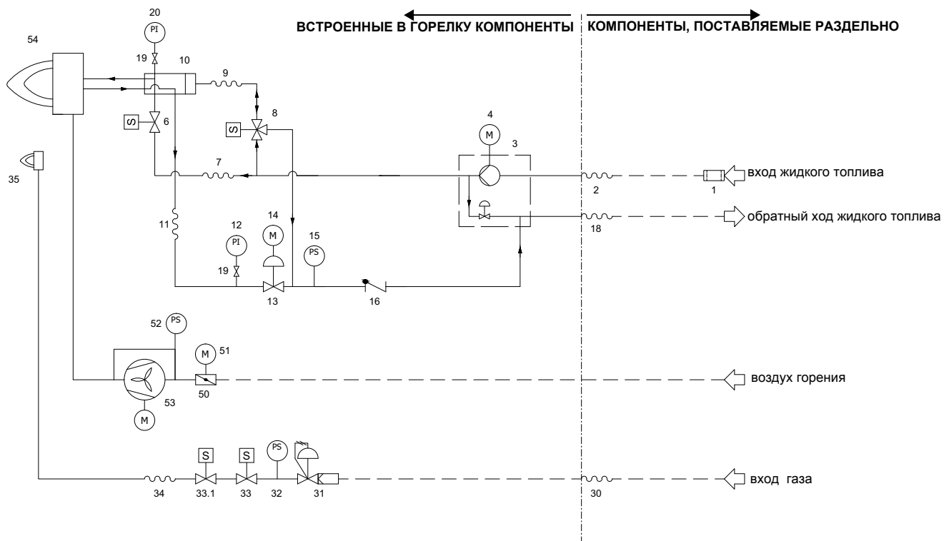
Рис. 2 - 3I2G-27 v0 – Гидравлическая схема для форсунки типа M3
