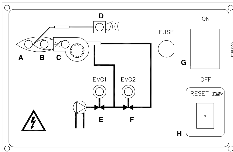
Fig. 20 - Bruciatori Bistadio
