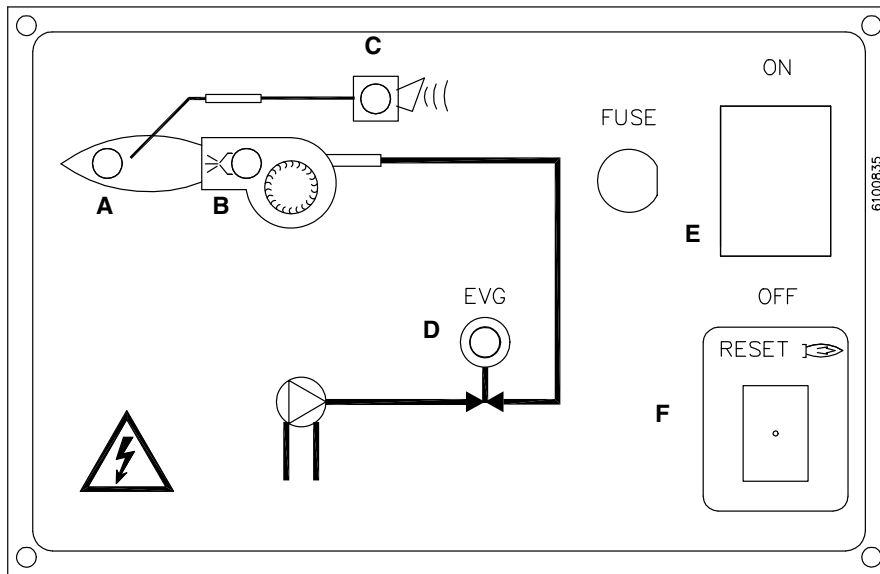
Fig. 19 - Bruciatori monostadio
