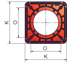
Фланец горелки
