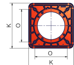
Flangia bruciatore
