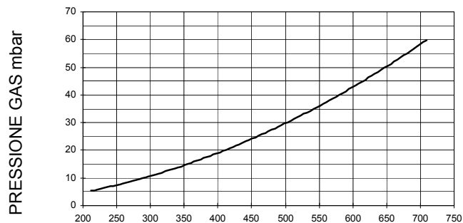
HR525A MG.. Rp2
