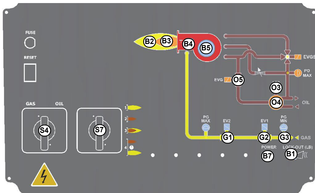
Fig. 5 - Pannello frontale quadro elettrico bruciatore
