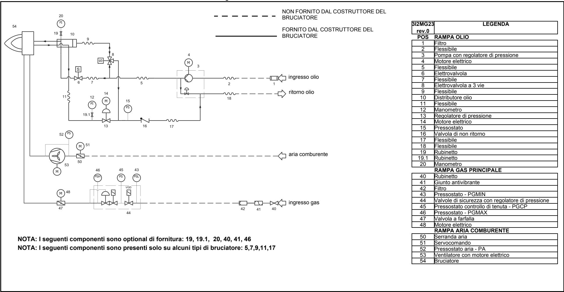
Fig. 2 - 3I2MG-23 v0 Schema idraulico
