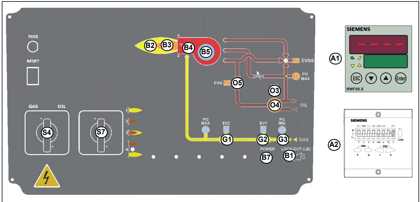
Рис. 11: передняя панель электроцита горелки
