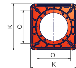
Flangia bruciatore
