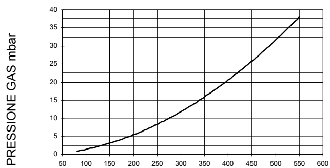
HR515A MG..
