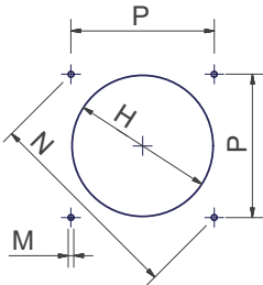
Plantilla de perforación de la placa de la caldera.
