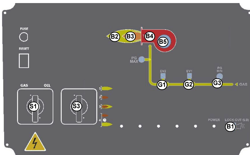
Fig. 4 Panel frontal cuadro eléctrico
