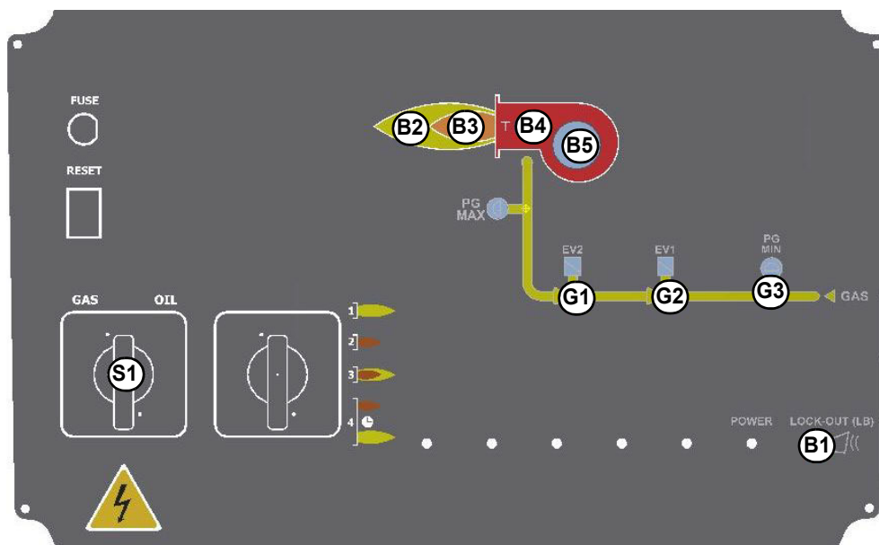
Fig. 5 - Pannello frontale quadro elettrico bruciatore
