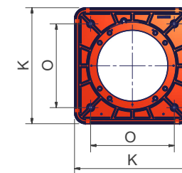
Flangia bruciatore
