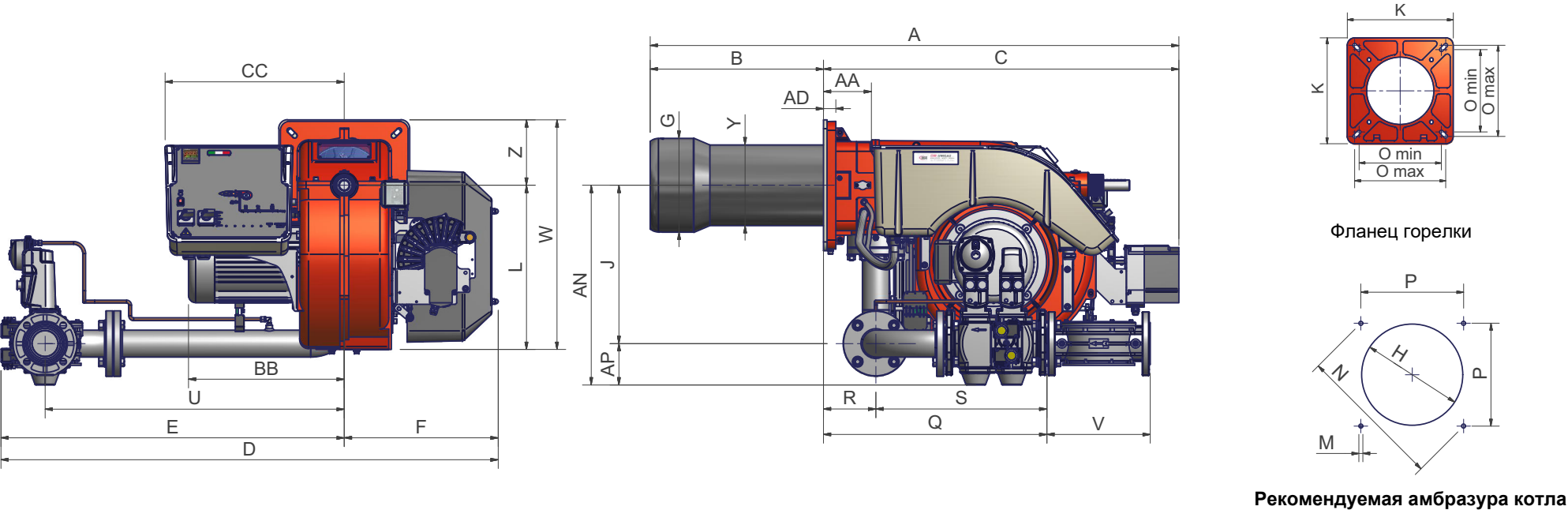
Рекомендуемая амбразура котла
