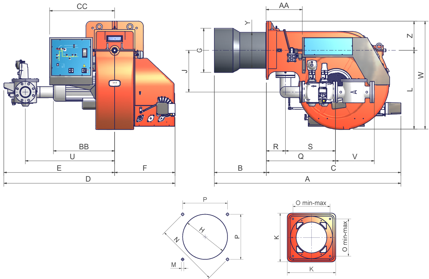
рекомендуемое исполнение амбразуры котла - фланцы горелок
