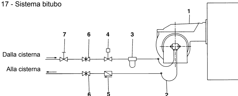
Fig. 17 - Sistema bitubo
