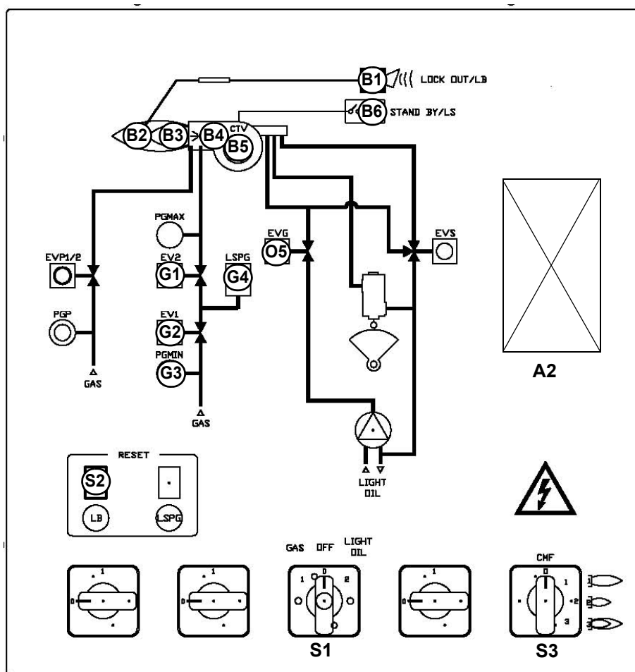
Fig. 12 - Pannello quadro elettrico
