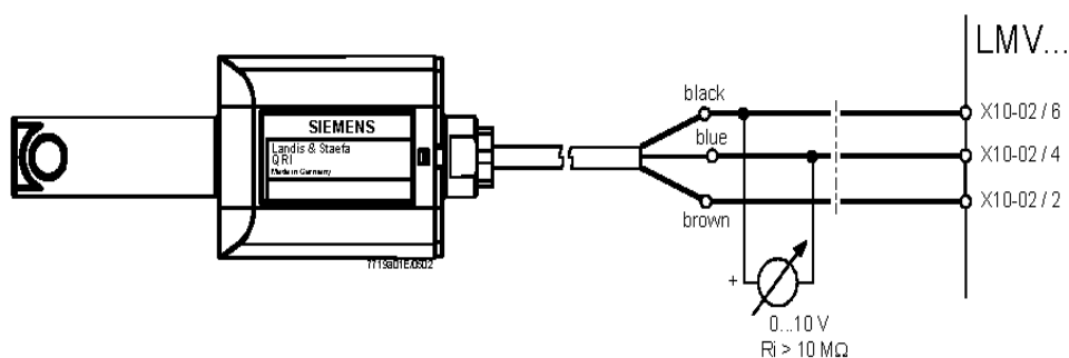
Fig. 22 - Rilevazione con fotocellula QRI..
