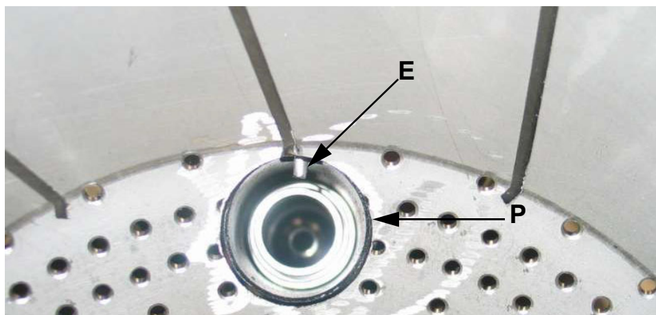
Fig. 20 - Particolare del diffusore con pilota (P) e elettrodo di accensione (E)
