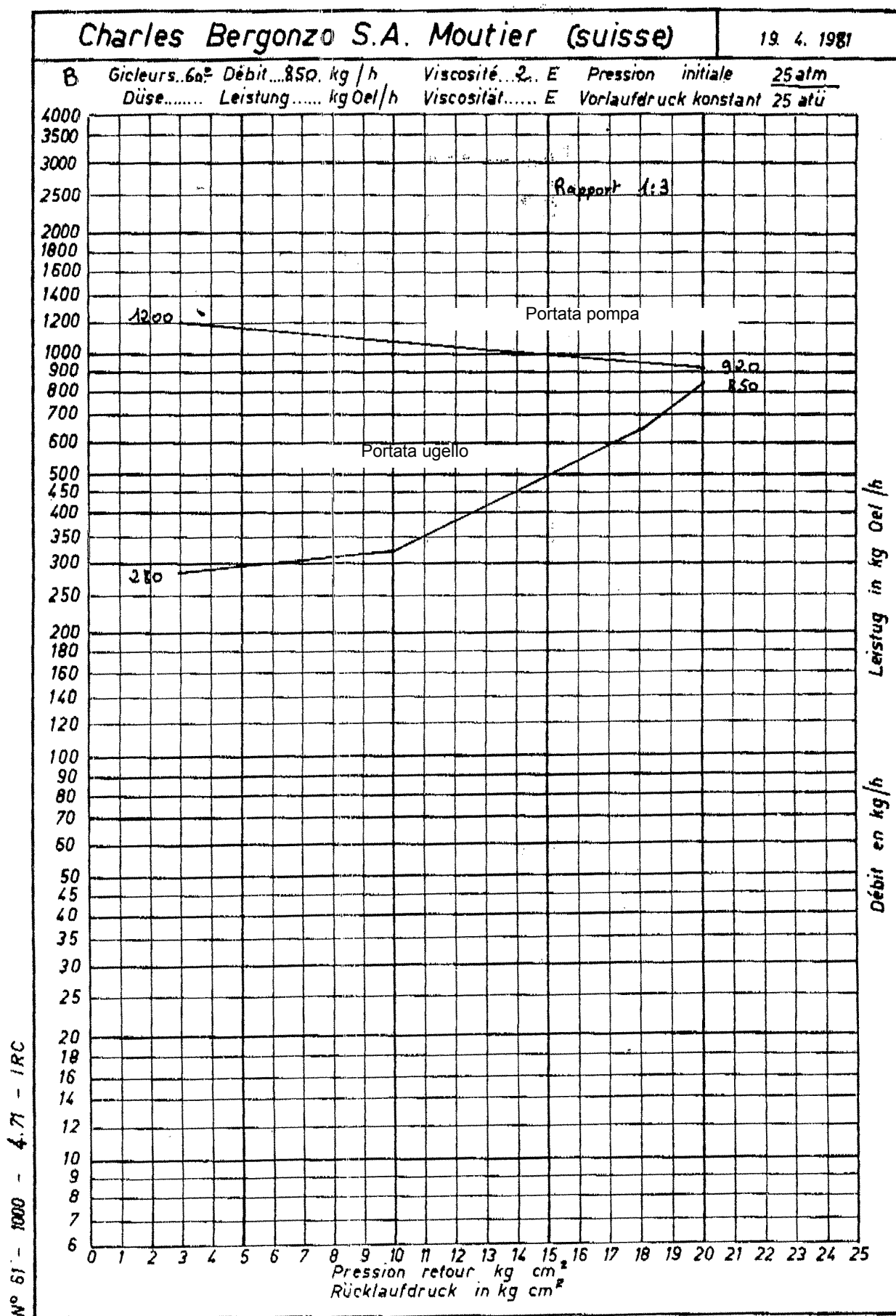
Fig. 16 - Ugello Bergonzo B- Esempio con ugello da 850 kg/h
