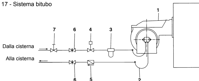
Fig. 17 - Sistema bitubo
