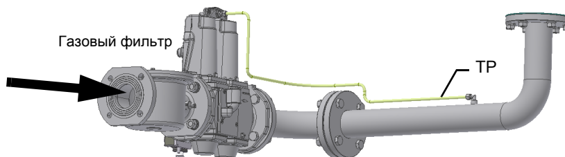
Siemens VGD... со SKPx Пример газовой рампы
