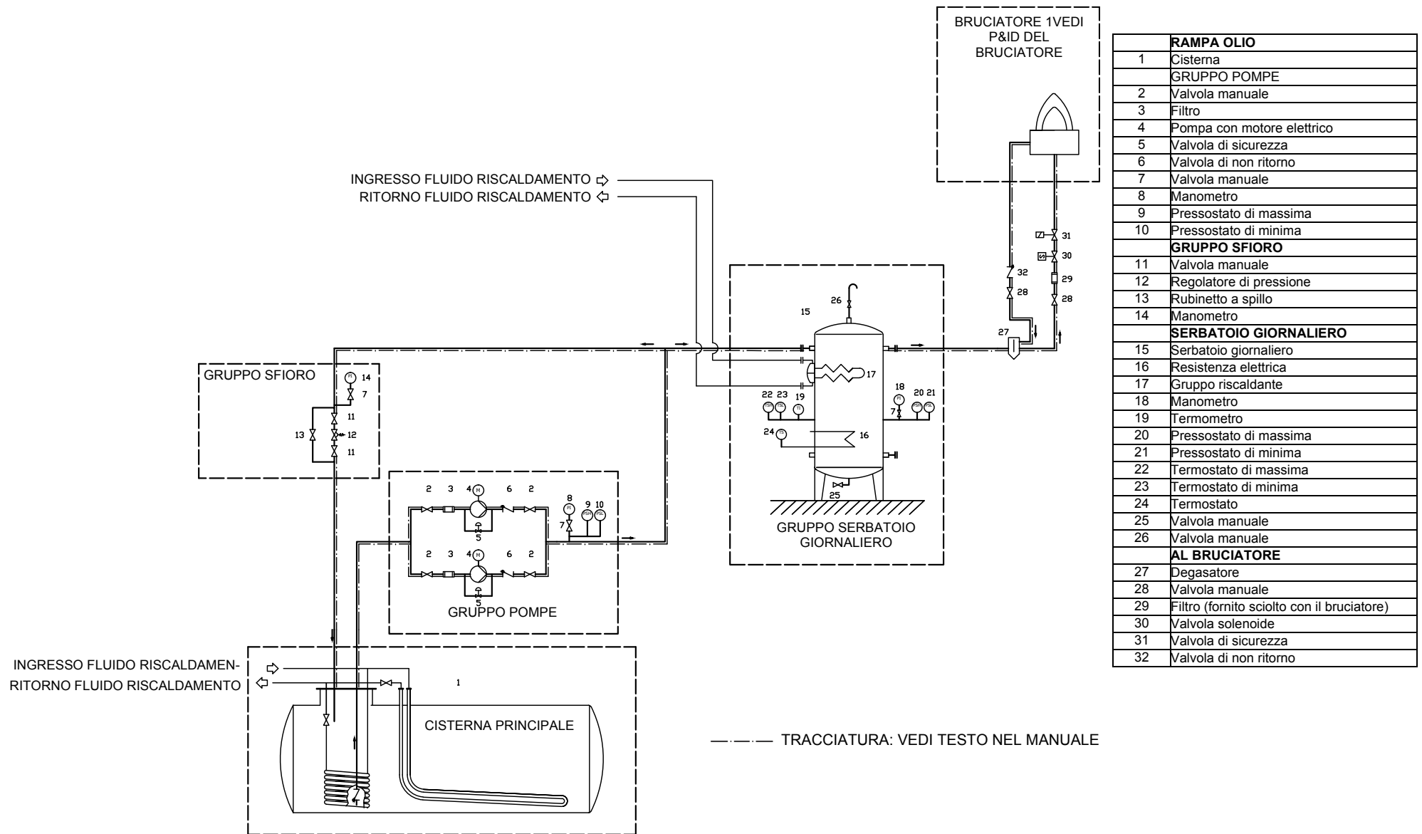
Fig. 18 - 3ID0023 v2 - Schema idraulico - Configurazione per un solo bruciatore
