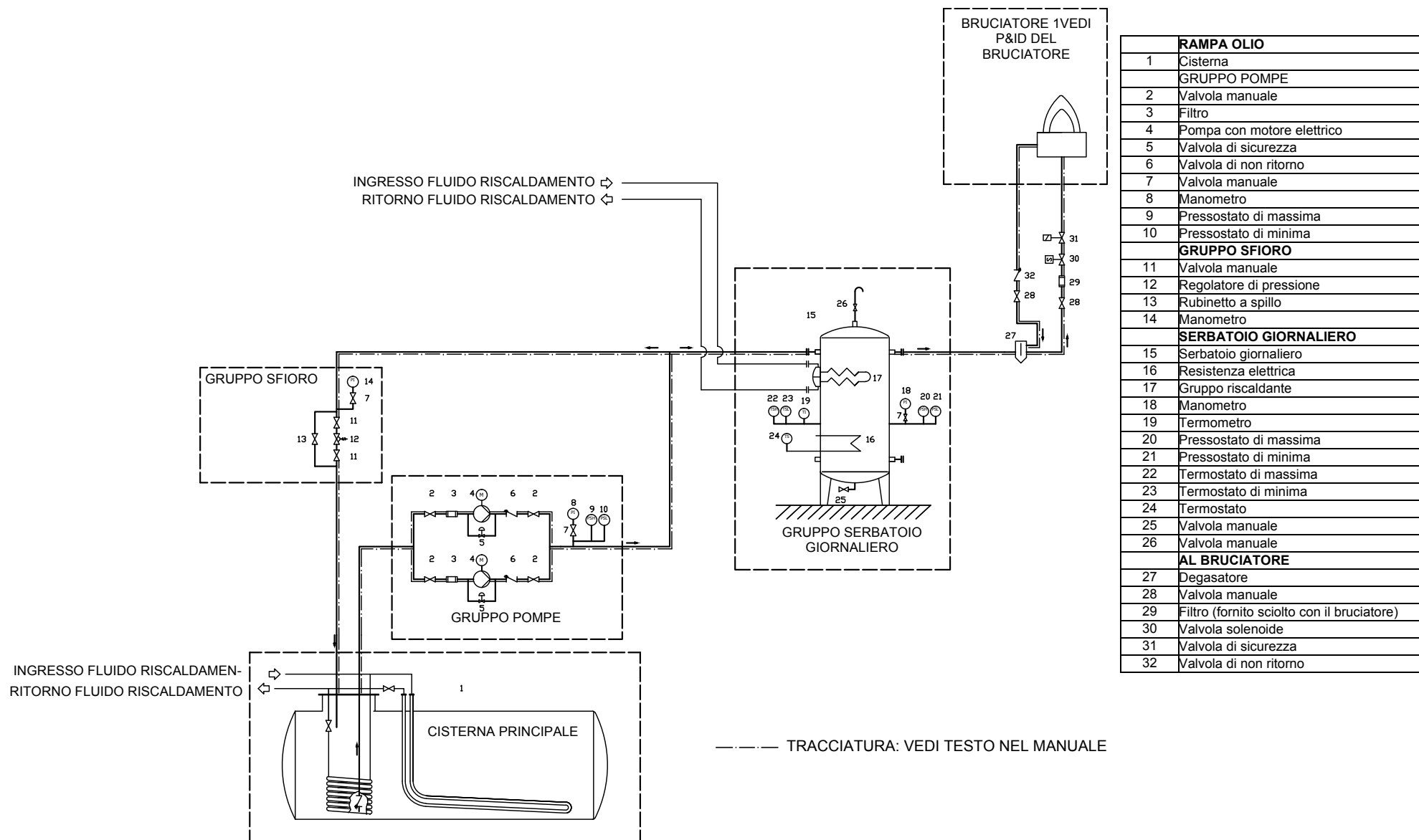
Fig. 18 - 3ID0023 v2 - Schema idraulico - Configurazione per un solo bruciatore
