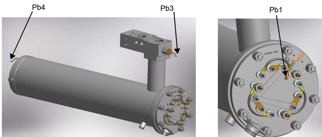
Fig. 18 - Collegamenti sonde Danfoss MCX (per bruciatori con 1 barilotti)
