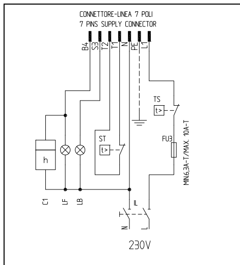
Fig. 32 - Connettore 7 poli
