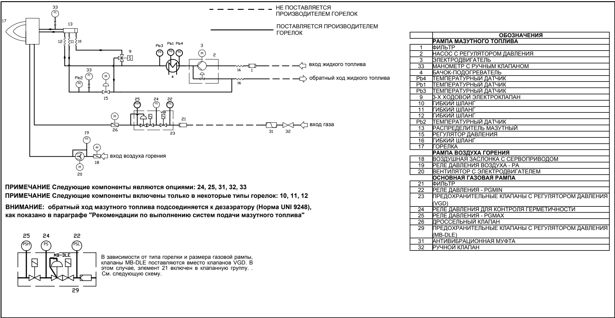
Рис. 1 Гидравлическая схема (3I2MD22 v1)
