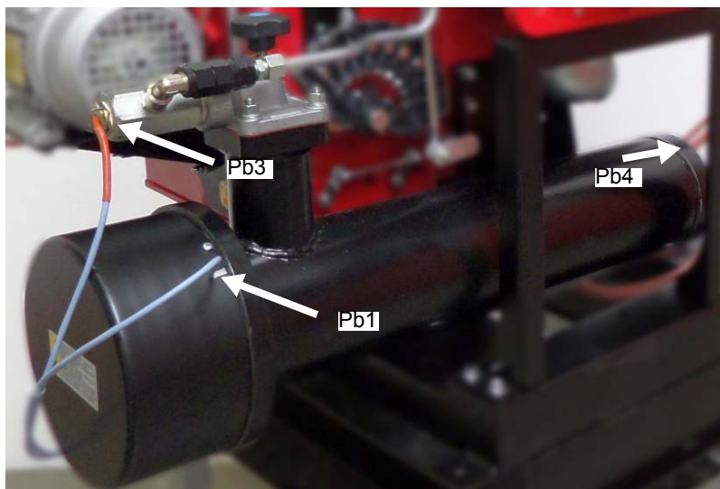
Рис. 30 Подключение датчиков DANFOSS MCX
