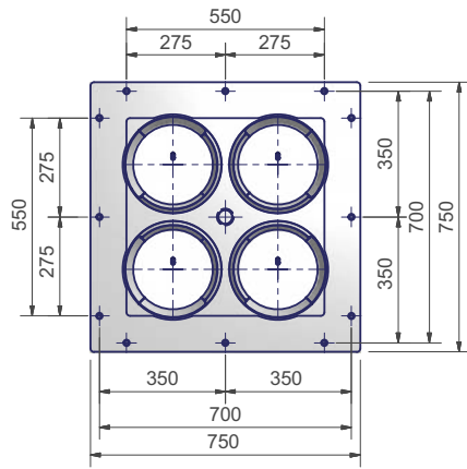
Фланец горелки
