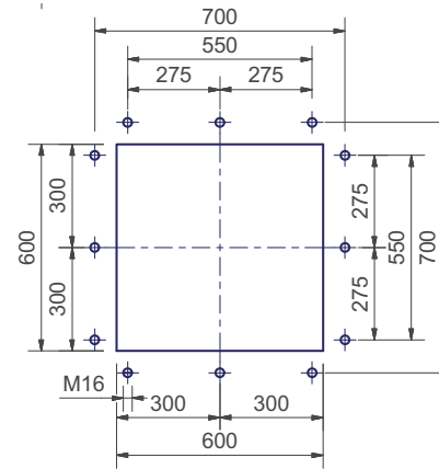
Рекомендуемая амбразура котла
