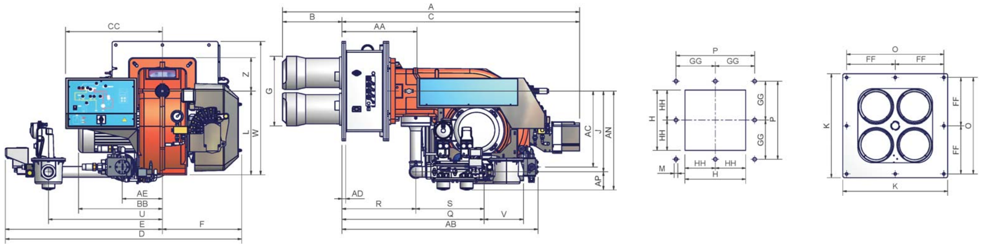
Рекомендуемая амбразура котла и фланцы горелок
