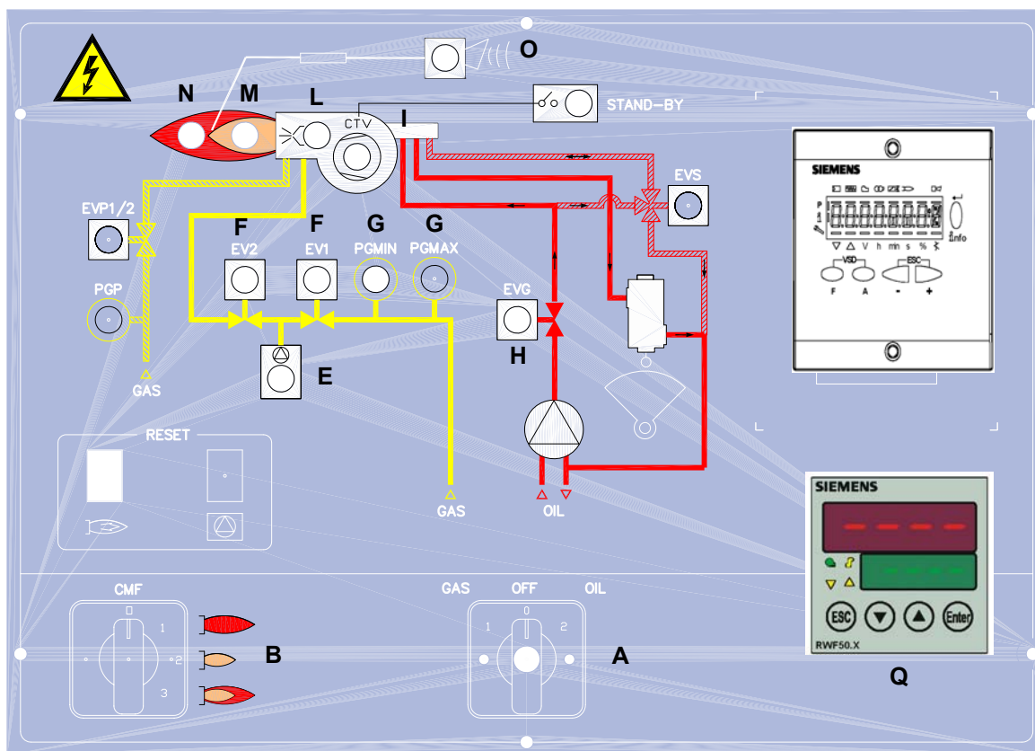
Рис. 22 Лицевая панель электрощита
