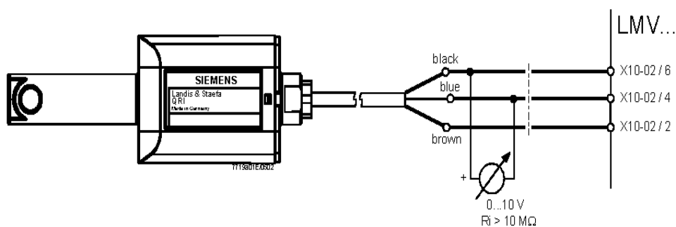
Рис. 31 - Детектирование с фотоэлементом QRI..
