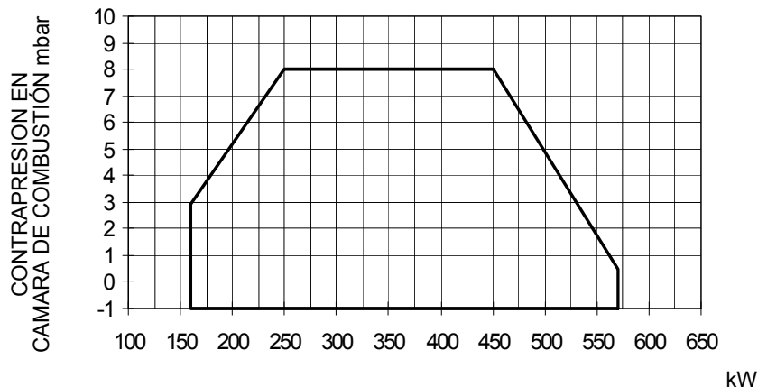
NGX550 Quemadores de baja emisión de NOx
