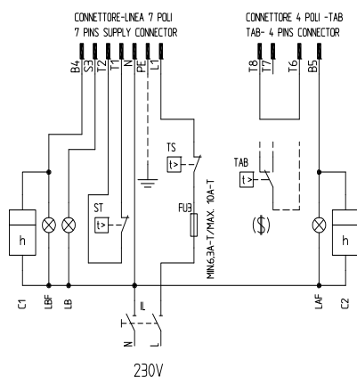
Fig. 16 - Conectores 7 y 4 polos
