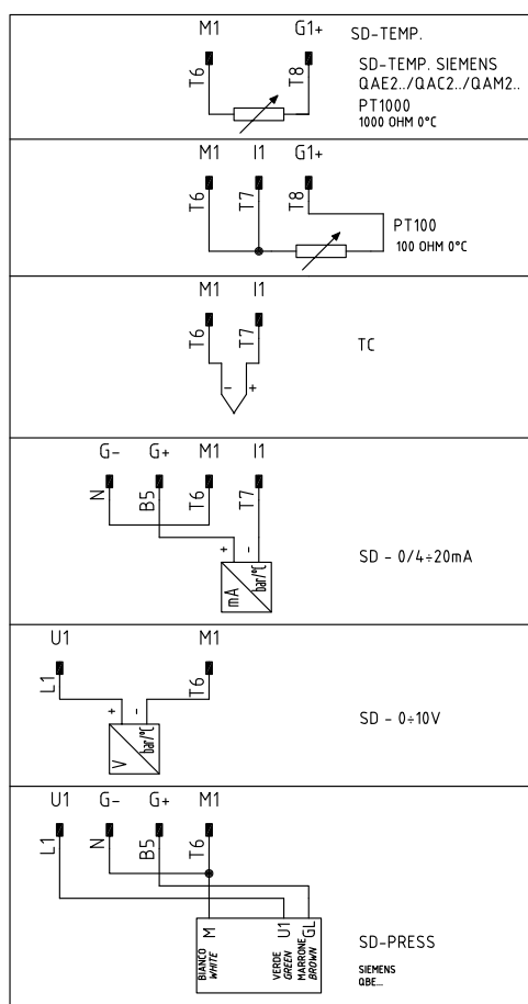
Fig. 18 - Conexión de las sondas
