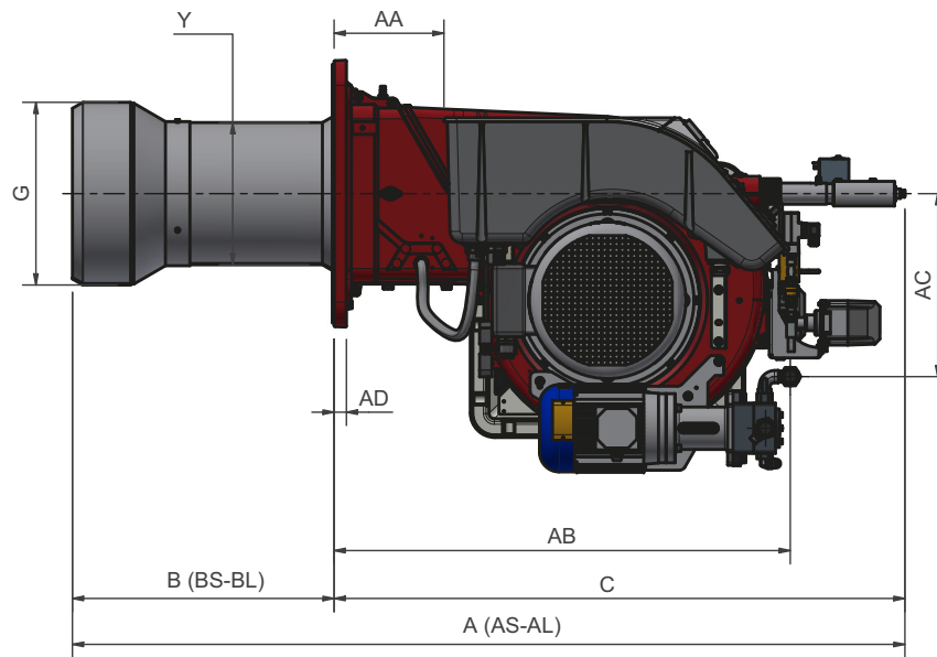
Фланец горелки
