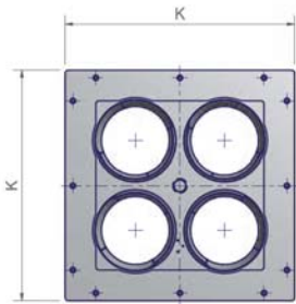
Flangia bruciatore
