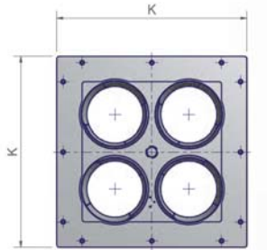
Flangia bruciatore
