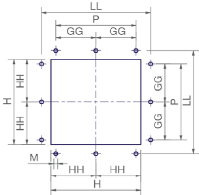
Foratura caldaia
