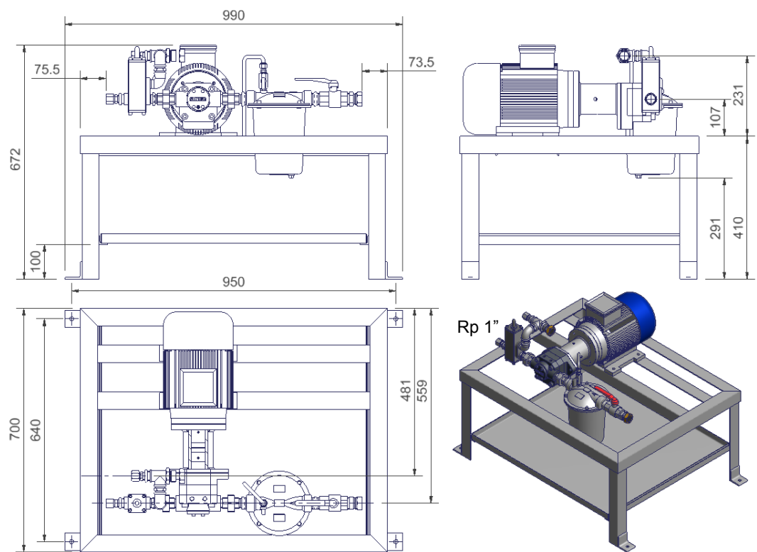
Fig. 5 Dimensioni di ingombro massimo del gruppo spinta (taglia bruciatore, da 525. Motore pompa ≥ 4kW)
