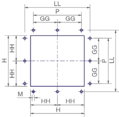
Foratura caldaia
