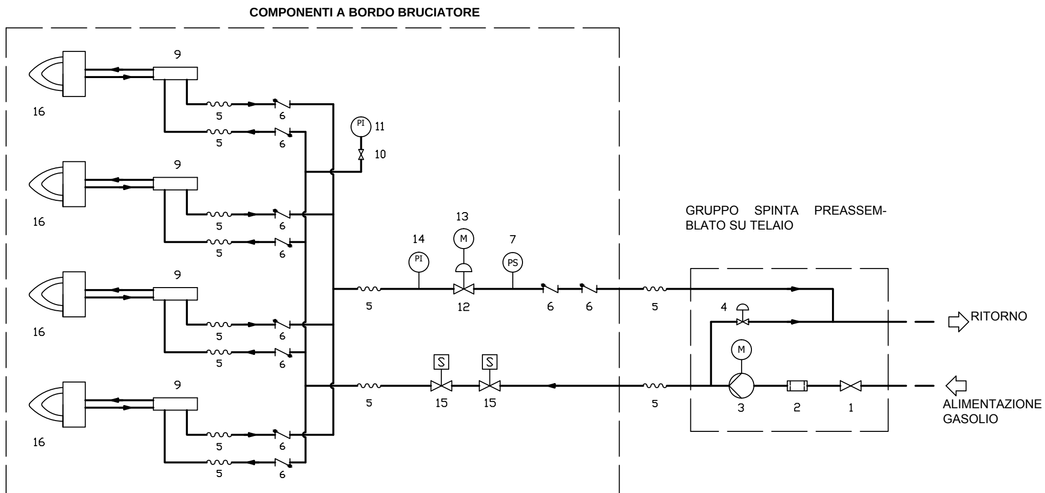
Fig. 7 Schema idraulico bruciatore (variante 2)
