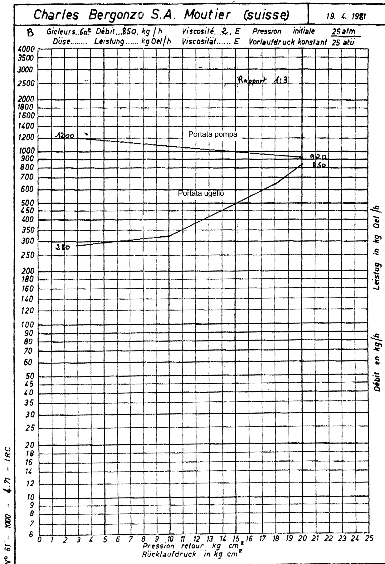
Fig. 23 - Ugello Bergonzo - Esempio con ugello da 850 kg/h
