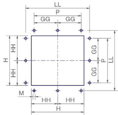
Foratura caldaia
