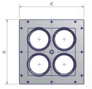
Flangia bruciatore
