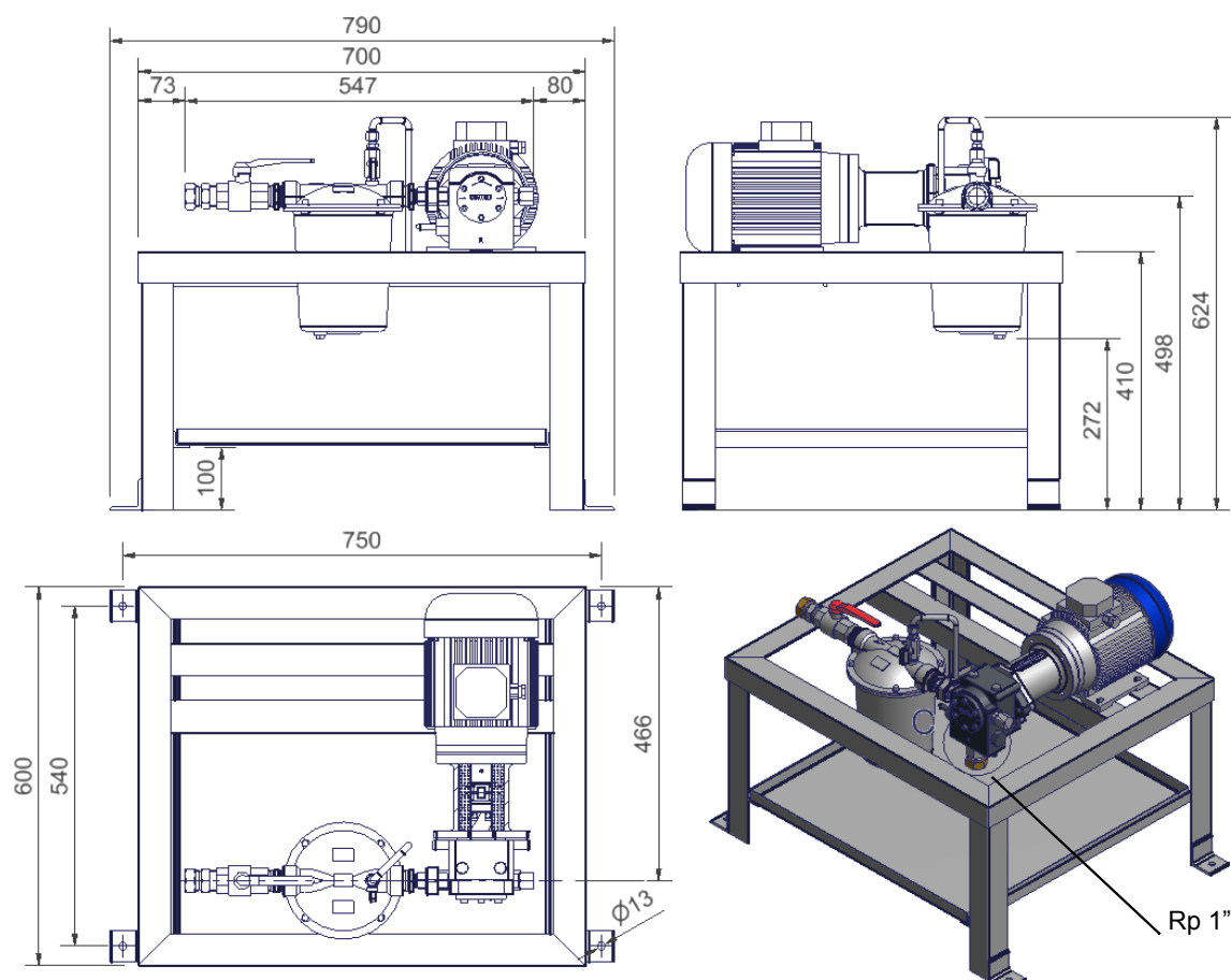
Fig. 4 Dimensioni di ingombro massimo del gruppo spinta (taglia bruciatore, fino a 520. Motore pompa &lt; 4kW)
