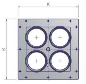
Flangia bruciatore
