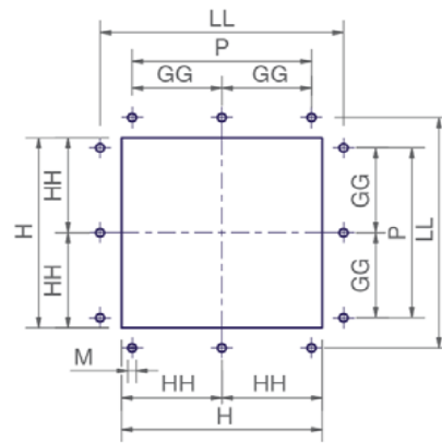
Foratura caldaia
