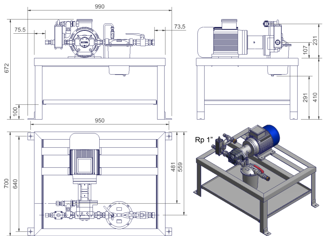
Fig. 5 Dimensioni di ingombro massimo del gruppo spinta (taglia bruciatore, da 525. Motore pompa \geq 4 kW)
