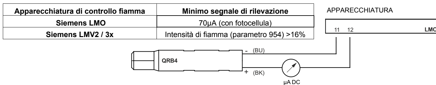
Fig. 1: Rilevazione con fotocellula QRB4
