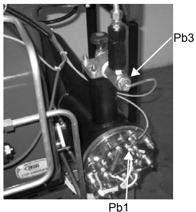
Fig. 15 - Collegamenti sonde Danfoss MCX
