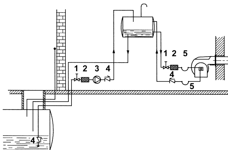
Рис. 9 - Контур подачи топлива под силой гравитации
