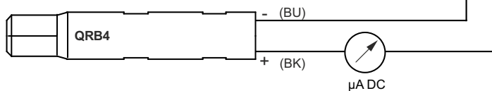
Fig. 1: Rilevazione con fotocellula QRB4
