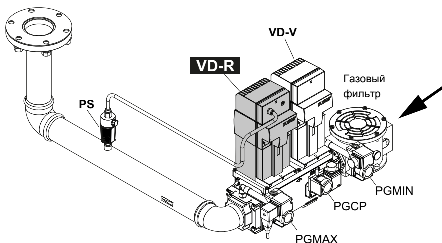
Рис. 7 - Пример газовой рампы
