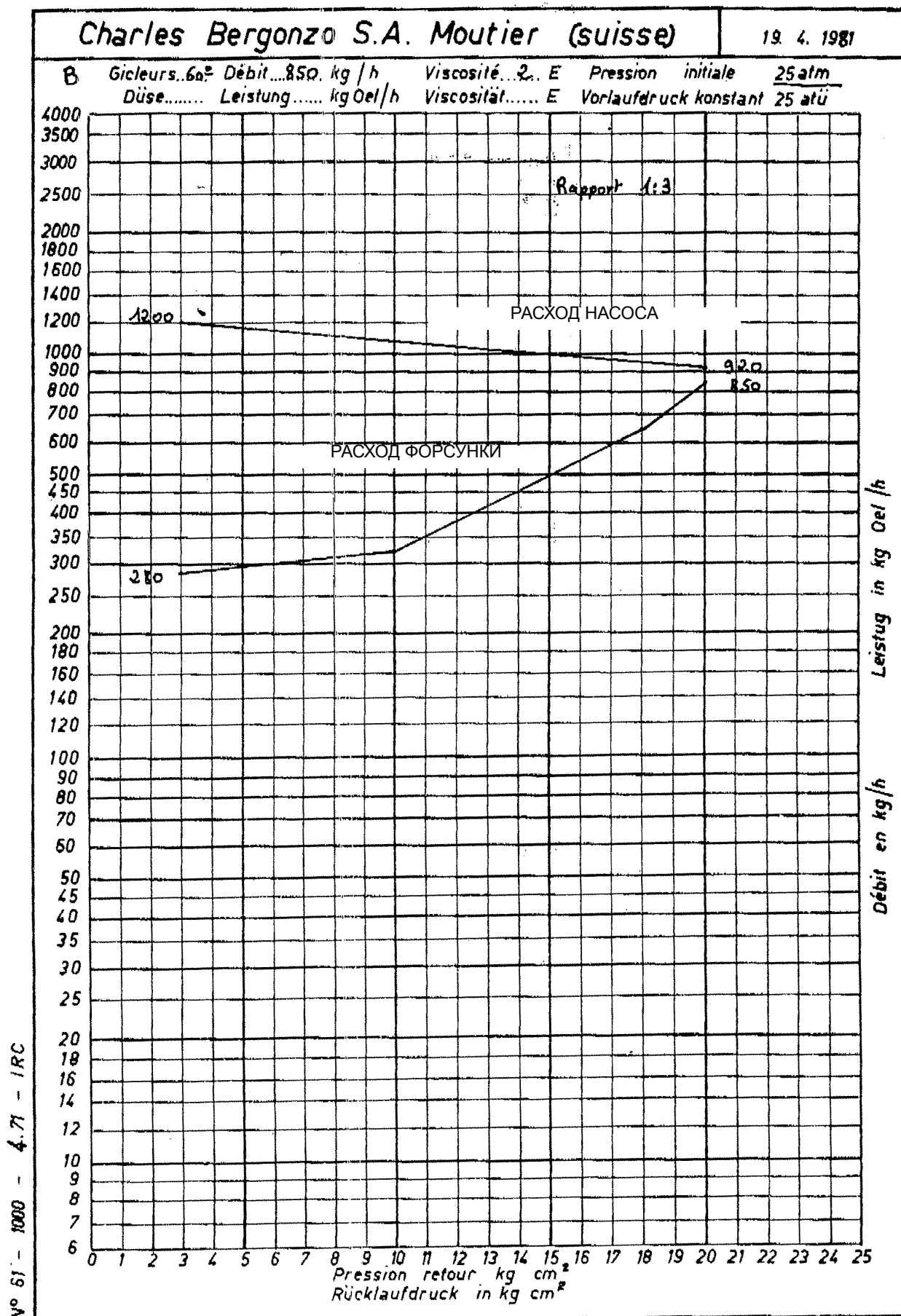
Рис. 16 - ФОРСУНКА BERGONZO B - Пример с форсункой с расходом 850 кг/час
