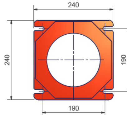
FLANGIA BRUCIATORE BURNER FLANGE
