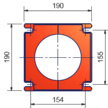
FLANGIA BRUCIATORE BURNER FLANGE
