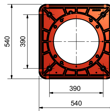
Фланец горелки
