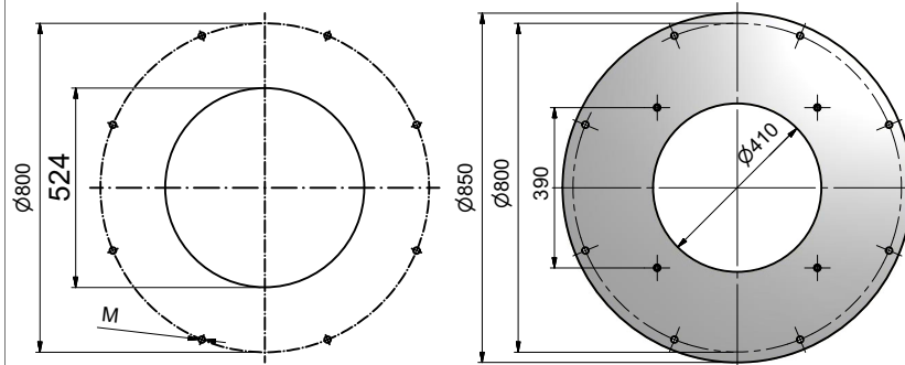
Рекомендуемый контрфланец
