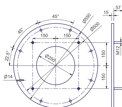
Рекомендуемый контрфланец
