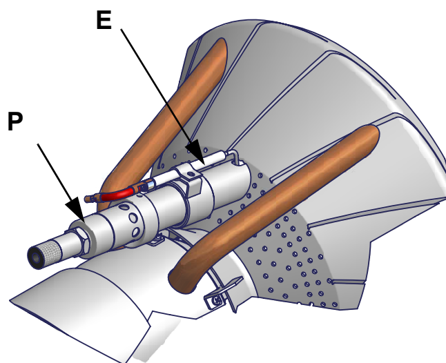
Fig. 11 - Particolare del diffusore con pilota (P) e elettrodo di accensione (E)
