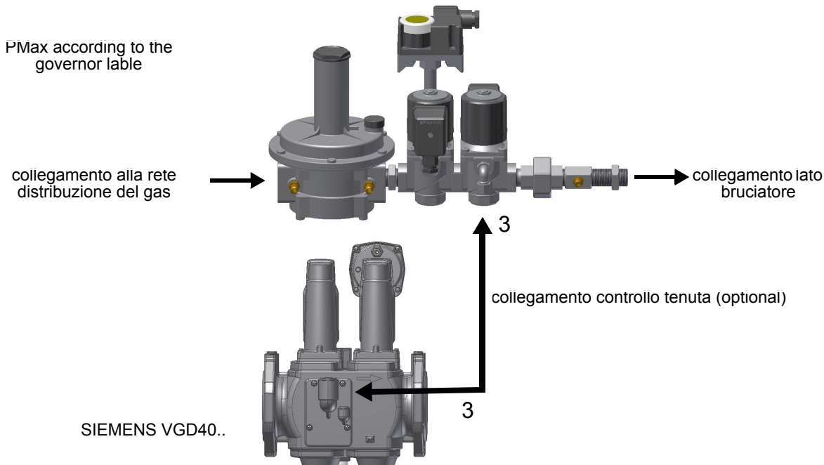
Fig. 5 - attacco (3) tubetto da rampa pilota al gruppo valvole della rampa principale (nello schema non è previsto ma si può eseguire)
