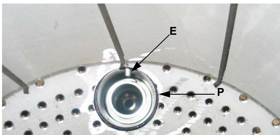
Fig. 11 - Particolare del diffusore con pilota (P) e elettrodo di accensione (E)
