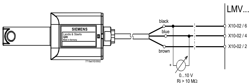
Рис. 11 - Детектирование с фотоэлементом QRI..
