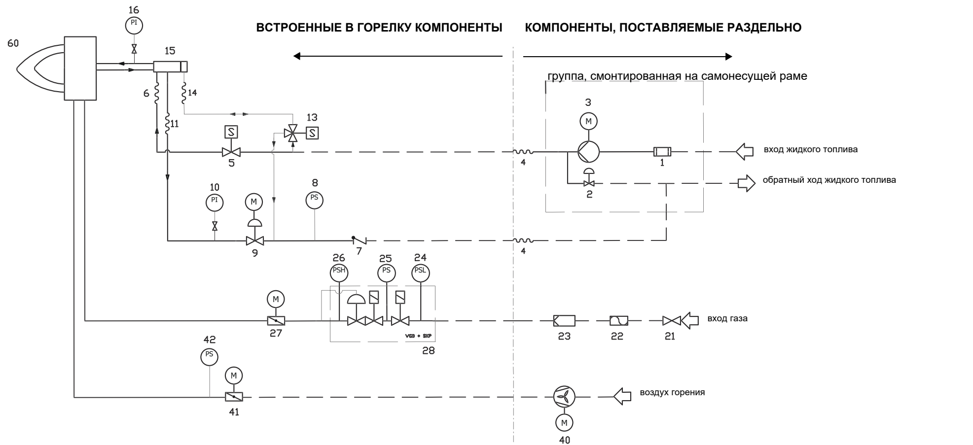
Рис. 4 Гидравлическая схема 3I2MG73 v0
