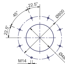
Foratura caldaia consigliata (HTP525A)
