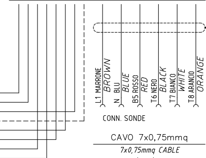
CAVO 7x0,75mmq 7x0,75mmq CABLE (xx)
