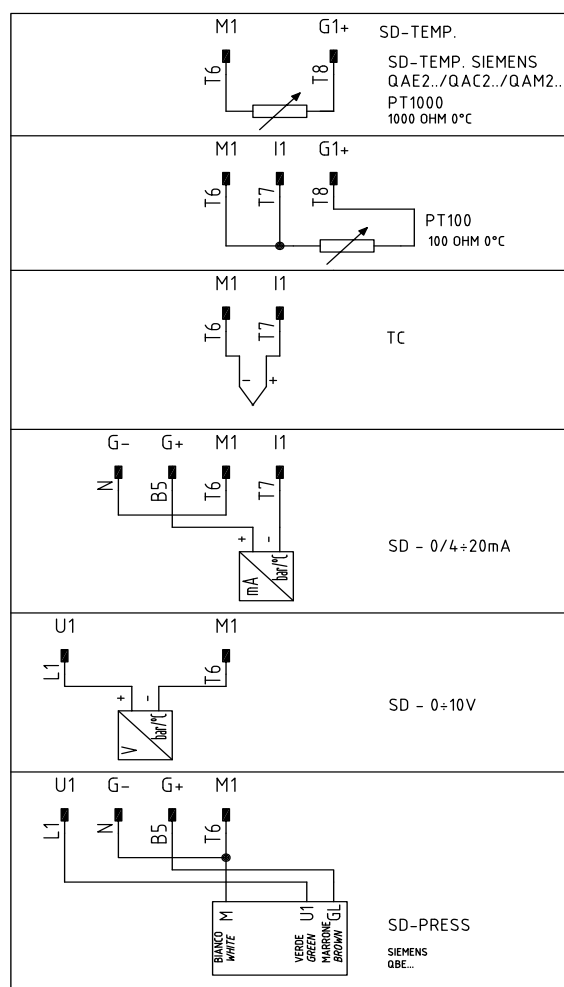
Fig. 34 - Collegamento sonda
