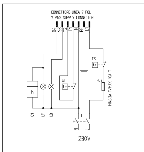
Fig. 32 Connettore 7 polii -
